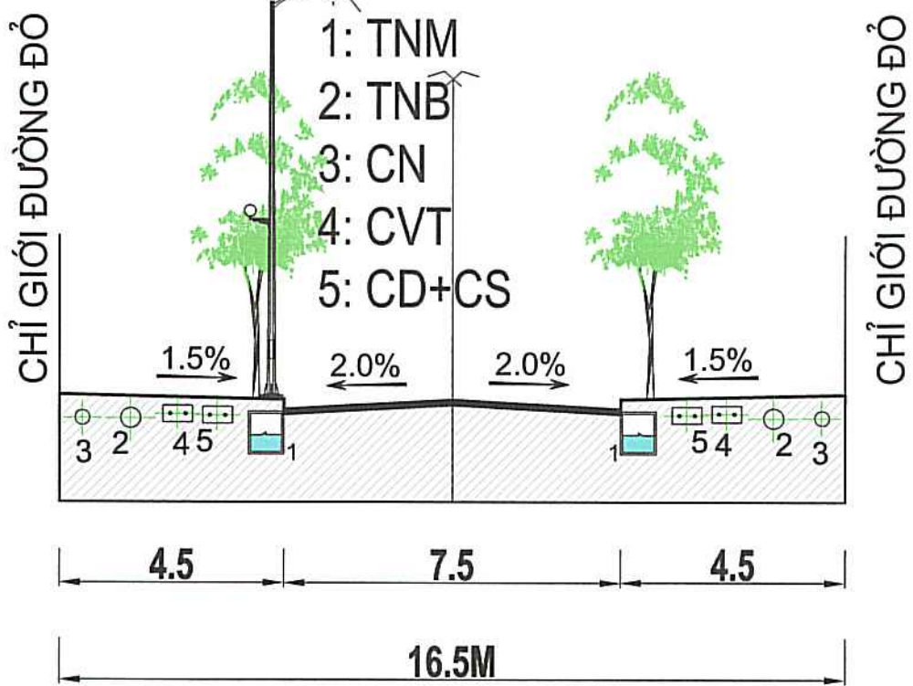
MẶT CẮT 1-1
