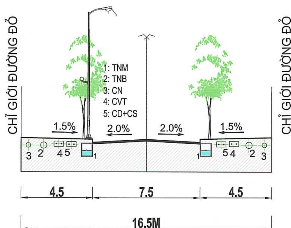
MẶT CẮT 1-1
