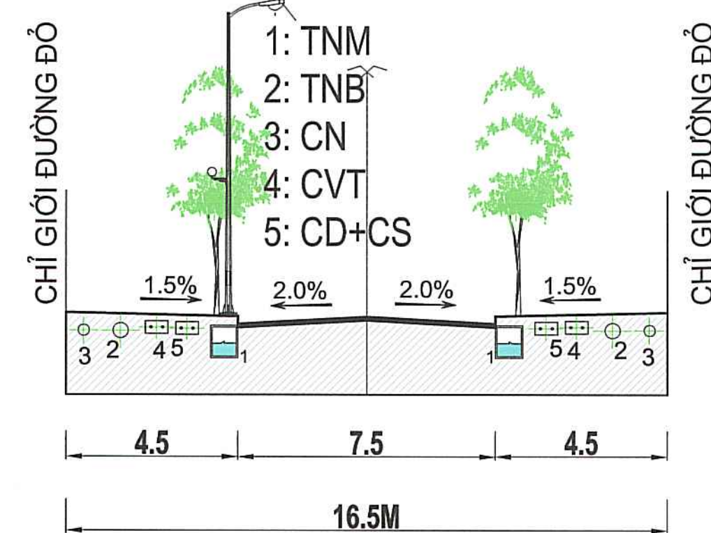
MẶT CẮT 1-1
