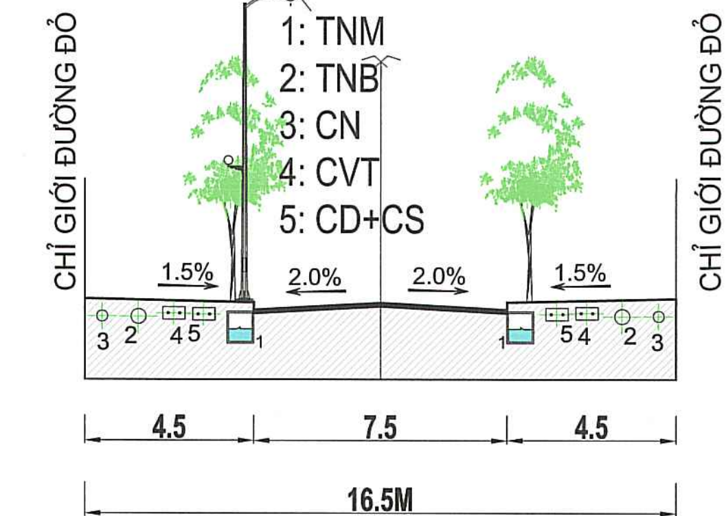
MẶT CẮT 1-1
